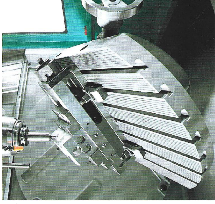
Due ulteriori assi di lavorazione grazie alla tavola rotante brandeggiabile manuale
